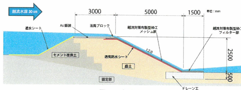
図-1 実験断面
