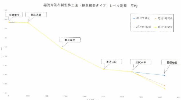
図-6 レベル計測結果（被覆工と基礎地盤の変位）
