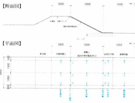
図-4 レベル計測位置
